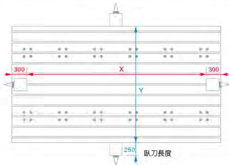
臥頭可加工尺寸 (工作台面積示意圖)
